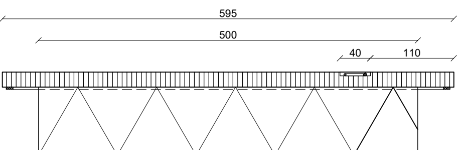
Doorsnede B-B
