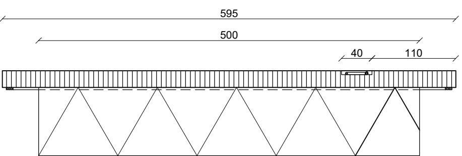
Doorsnede B-B
