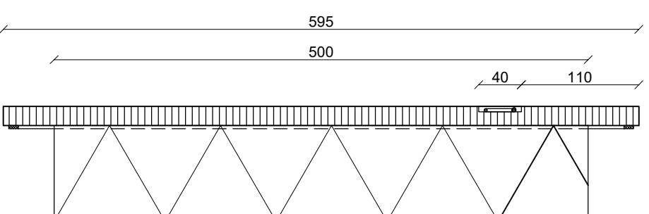
Doorsnede B-B
